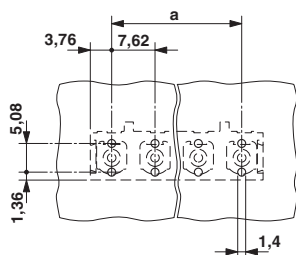
Vrtací schéma
